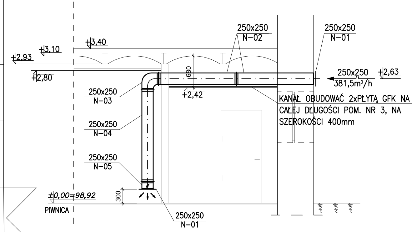
PRZEKRÓJ A-A x1:50x
